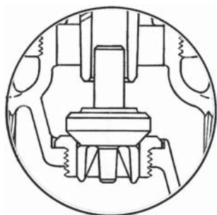
Figura 42: Disco cônico de aço inoxidável para válvulas de retenção horizontal Uso em fluidos agressivos e relativa sujeira
