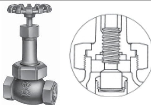
Figura 37: Válvulas Globo e Gaveta - Tampa acoplada ao corpo por meio de porca de união
