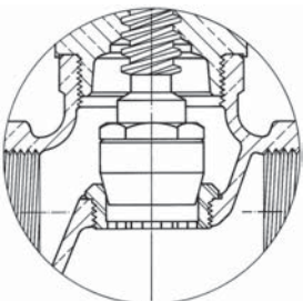
Figura 31 : Obturador para Válvula Globo Disco cônico tipo "plug" de aço inoxidável e sede postíça
