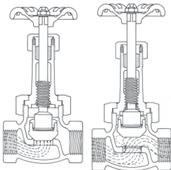
Figura 20: Válvulas Globo - Detalhes da forma do bloqueio do fluido e passagem em "S"
