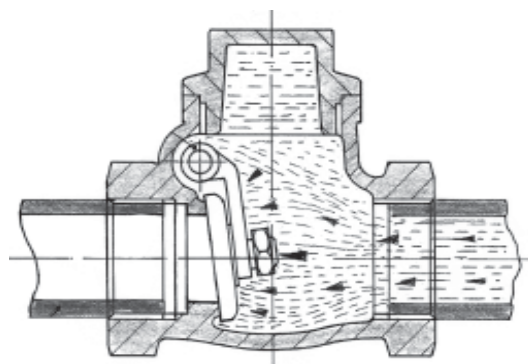
Figura 46: Válvula de retenção com portinhola Detalhe efeito retenção (bloqueio de refluxo)
