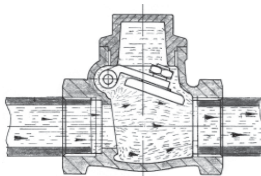
Figura 45: Válvula de retenção com portinhola Detalhe da passagem do fluido
