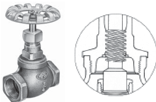
Figura 36: Válvulas Globo e Gaveta - Tampa acoplada diretamente ao corpo por meio de rosca interna
