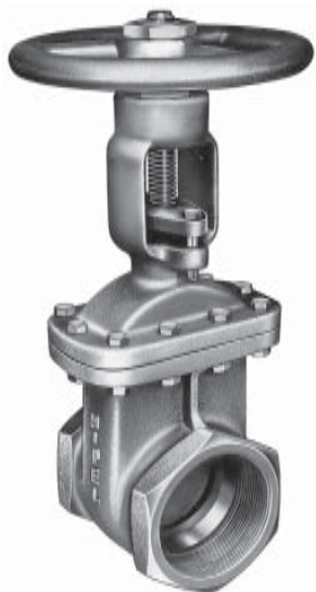
Figura 12: Válvula Gaveta com haste de rosca externa ascendente - Forma construtiva básica
