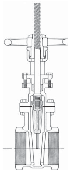
Figura 14: Válvula Gaveta com haste de rosca externa ascendente - Detalhe da distância centro a topo variável
