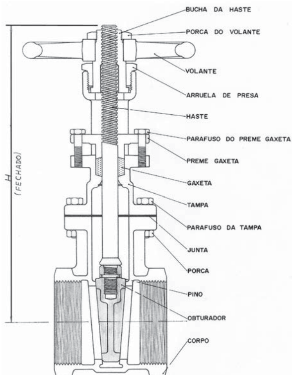
Figura 13: Válvula Gaveta com haste de rosca externa ascendente - Vista em corte
