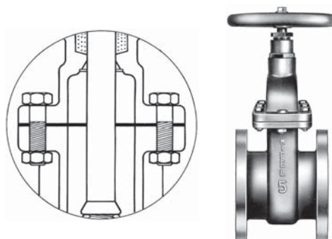
Figura 38: Válvulas Globo e Gaveta Tampa acoplada ao corpo por meio de parafusos
