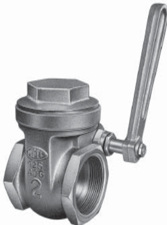
Figura 15: Válvula Gaveta de fecho rápido - Forma construtiva básica
