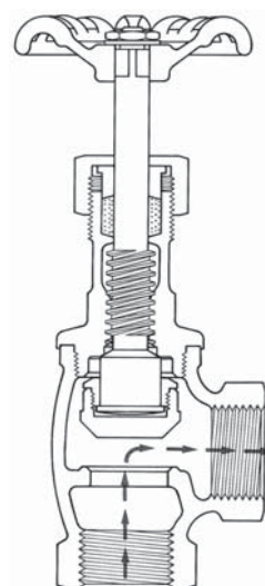
Figura 23: Válvula Angular - Detalhes da passagem do fluido e vedação
