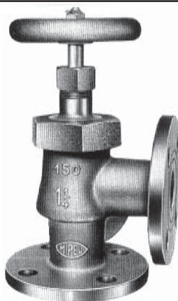
Figura 21: Válvula globo angular com extremidades flangeadas
