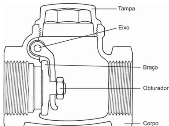
Figura 44: Válvula de retenção com portinhola Vista em corte
