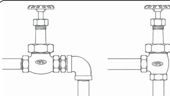
Figura 24: Válvulas globo reta e angular Detalhes típicos de instalação (na 1ª com uso de 4 junções, 1 niple e 1 cotovelo e na 2ª somente 2 junções)
